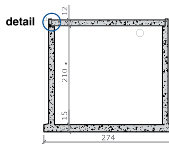
dwarse doorsnede coupe transversale
