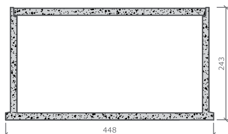
langse doorsnede coupe longitudinale
