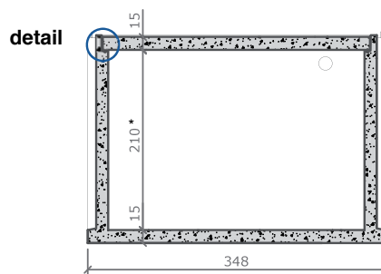
dwarse doorsnede coupe transversale
