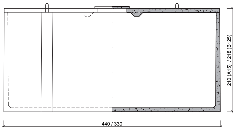
VOORAANZICHT / DOORSNEDE VUE FRONTALE / COUPE
